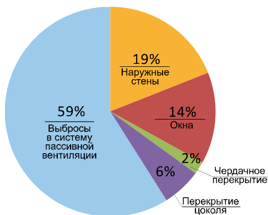
Рис. 11: Потери отпускаемой тепловой энергии в жилом типовом здании
